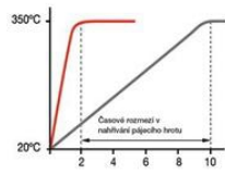
Průběh nahřívání hrotu
