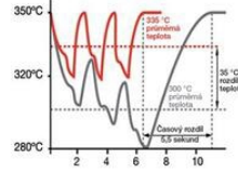
Průběh pájení
