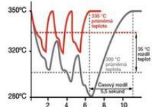
Průběh pájení
